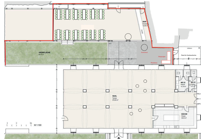
Tenne mit Tischen 70 x 220 cm Bereich A+B+C
